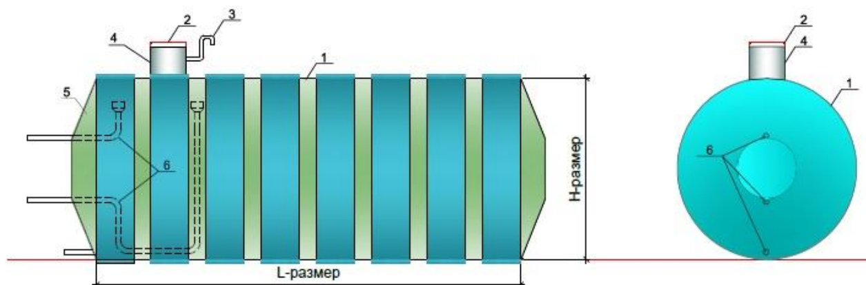
1 Корпус. 2 люк. 3 вентиляционный патрубок 4 горловина 5 торец резервуара. 6 система труб.
